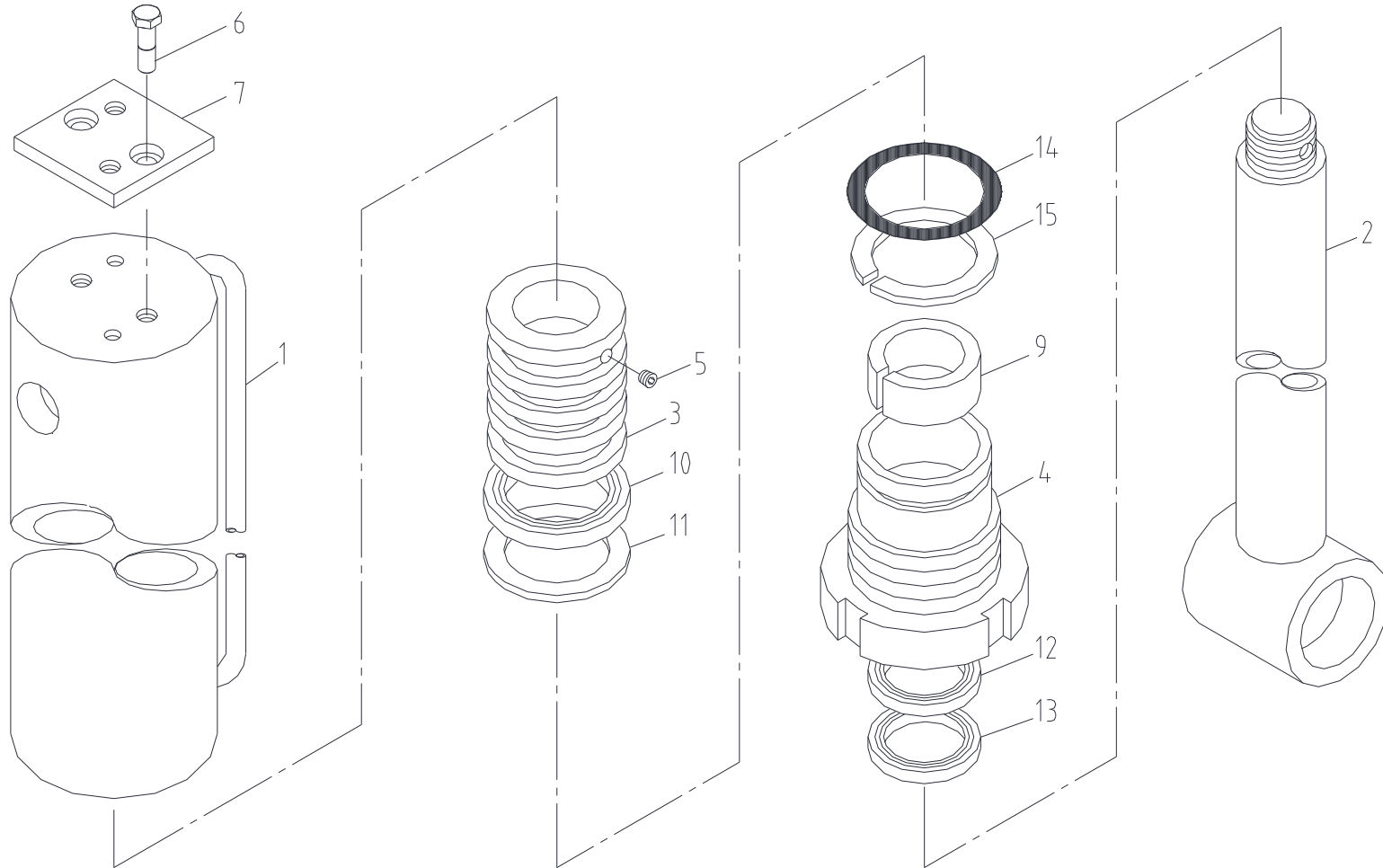
잭 실린더 조립체 Fig. 4-1 SCS513SL JACK CYL' ASS'Y
