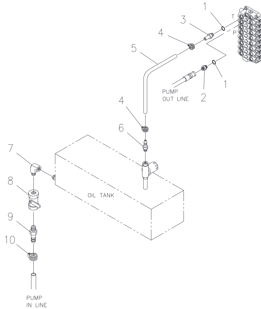
디스트리뷰터 배관 Fig. 5-1 SCS513SL DISTRIBUTOR PIPING
