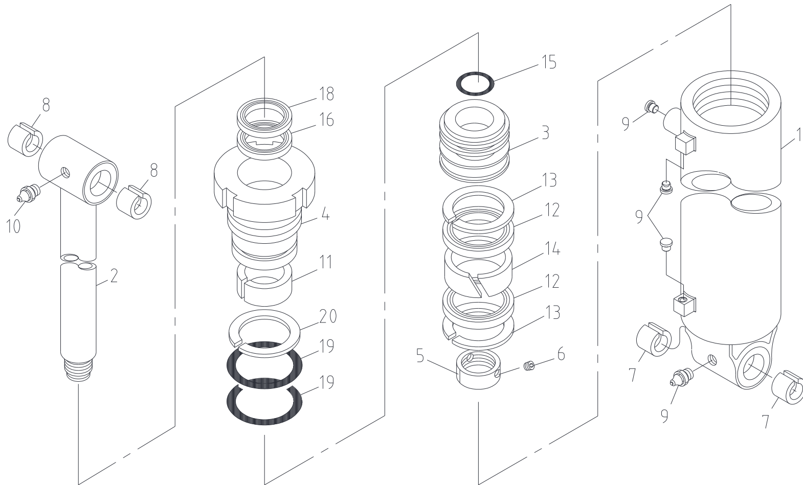
데릭 실린더 조립체 Fig. 2-3 SCS513SL DERRICK CYLINDER ASS'Y
