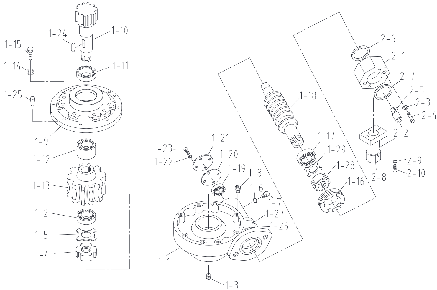
스윙 감속기 세트 Fig. 3-1 SCS513SL SWING R/ G SET
