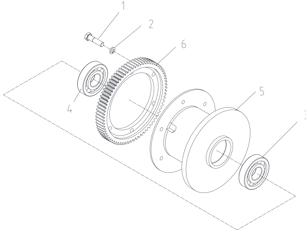
드럼 조립체 Fig. 2-1 SCS513SL DRUM ASS'Y
