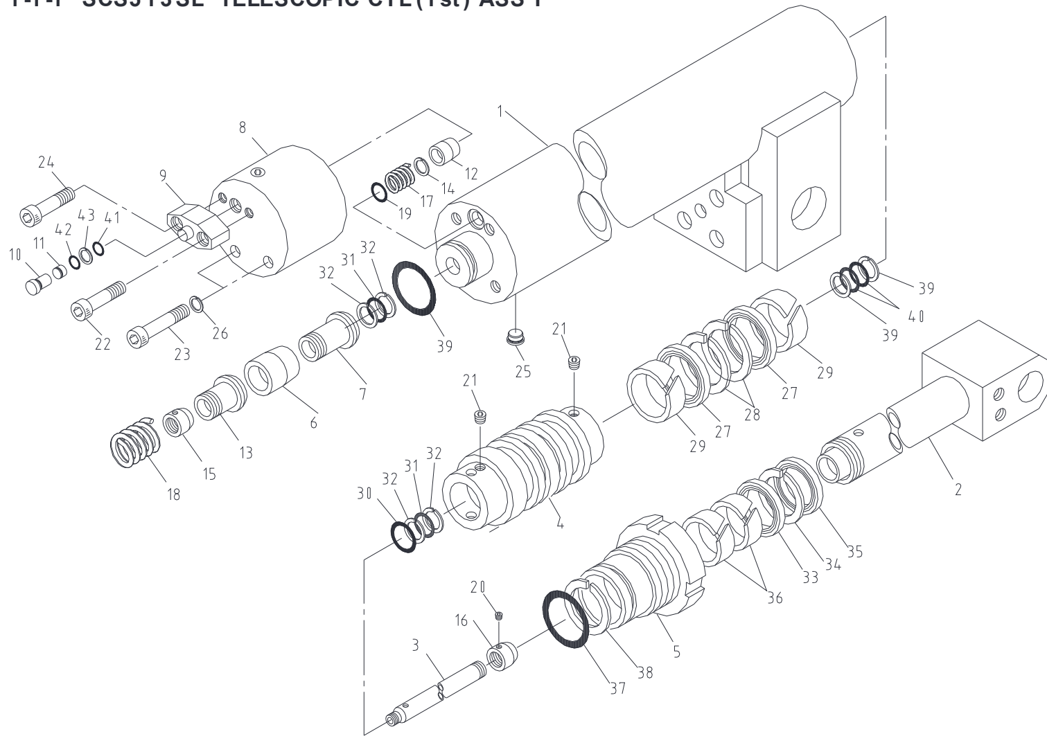
텔레스코픽 실린더(1 단) 조립체 Fig. 1-1-1 SCS513SL TELESCOPIC CYL'(1st) ASS'Y
