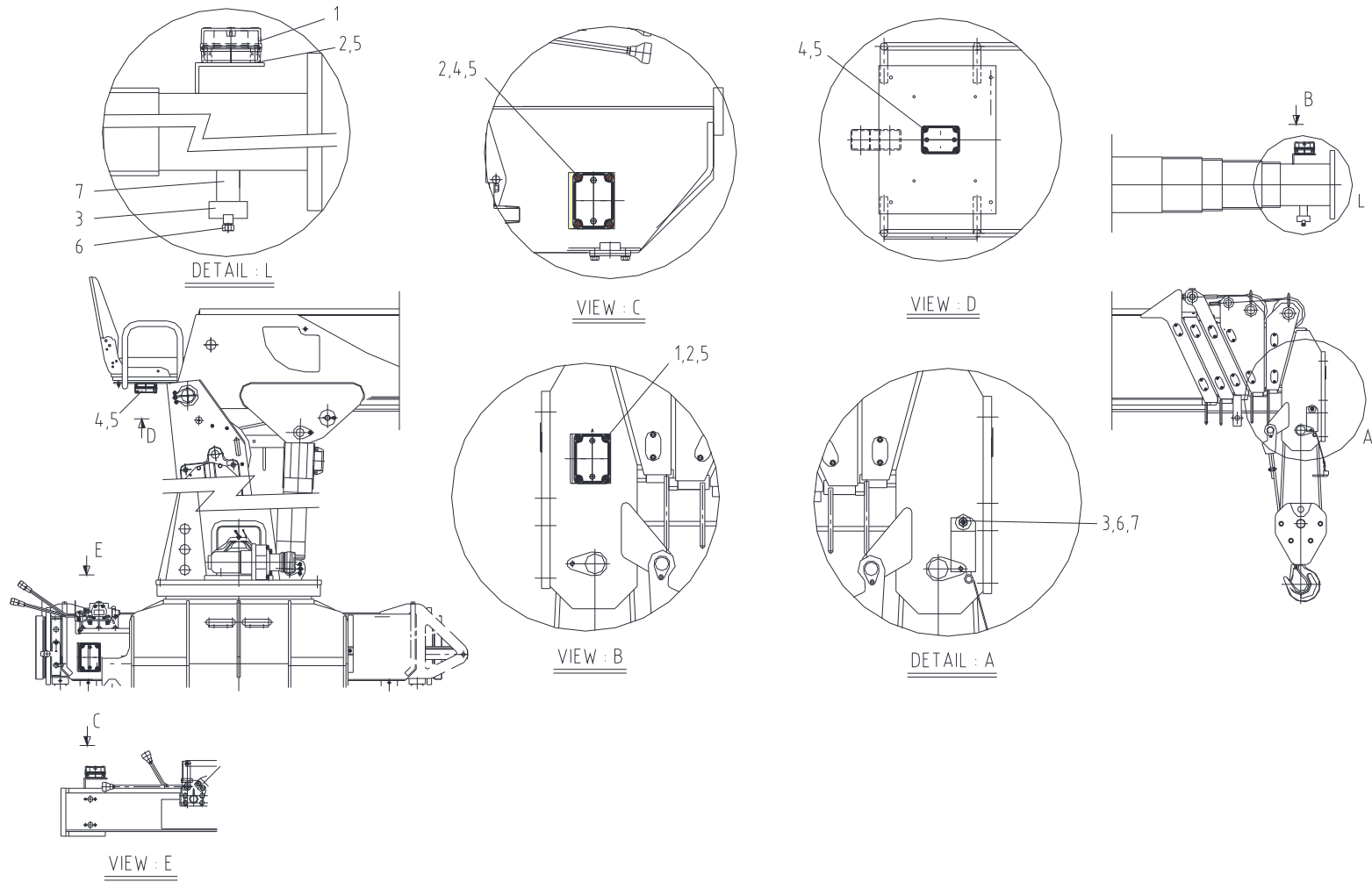
무선 과권 장치 위치도 Fig. 9-3-1 SCS513SL BOOM WIRING
