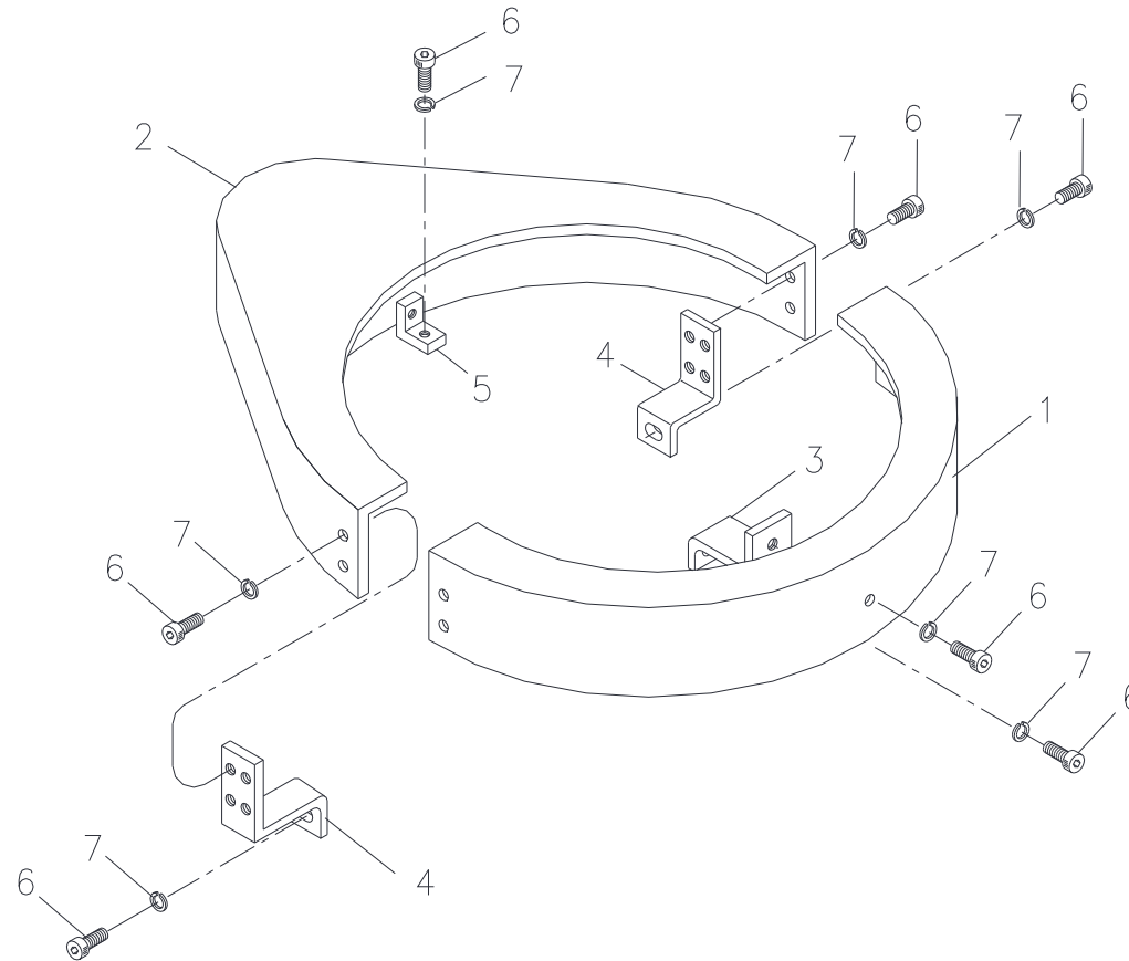
기어 커버 조립체 Fig. 3-5 SCS513SL GEAR COVER ASS'Y
